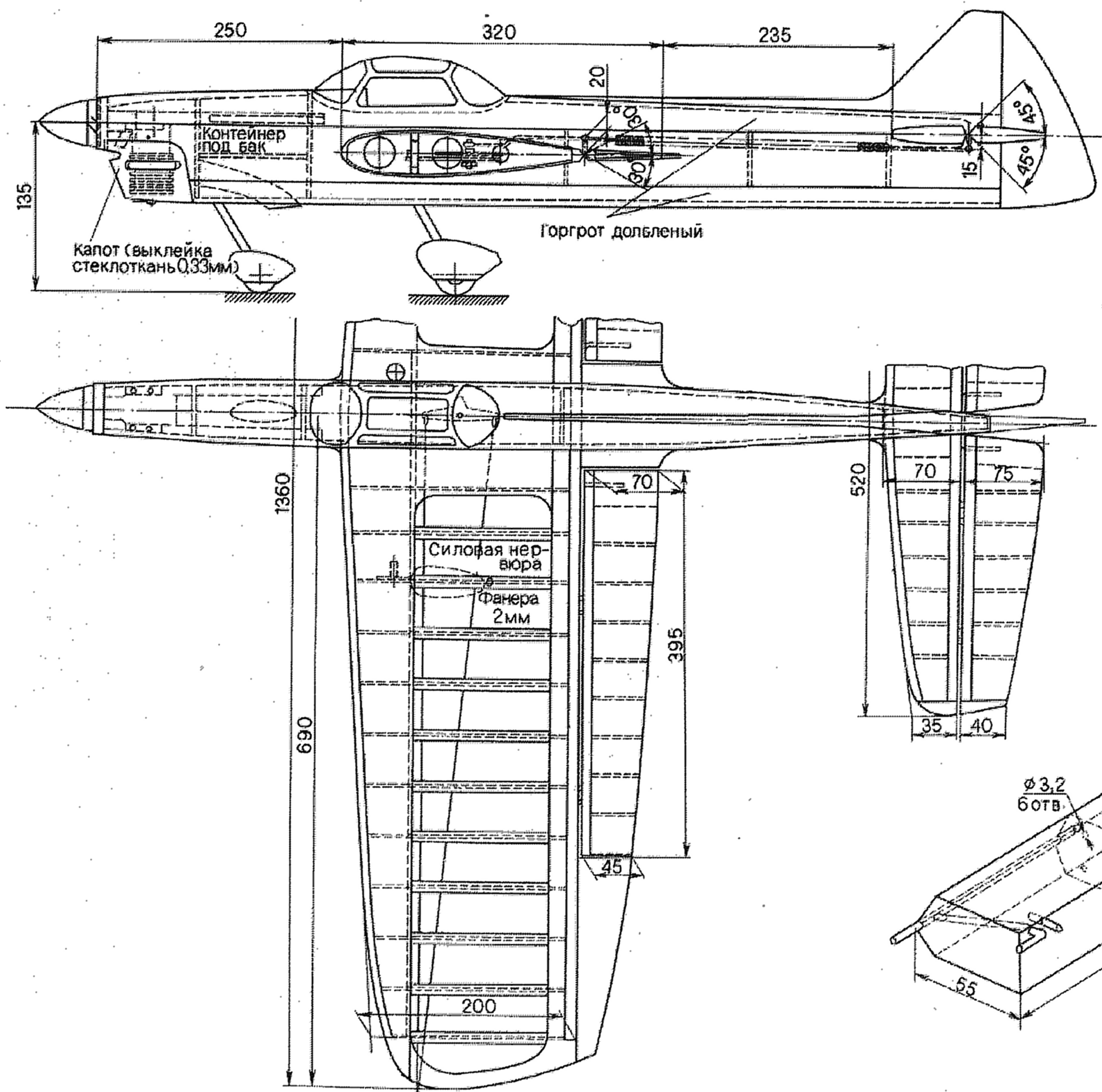
Чертеж модели мастера спорта СССР международного класса, чемпиона Украины, победителя международных соревнований, члена сборной команды СССР А. Крамских (Украина).
